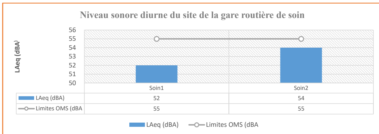
Figure 2: Résultat des mesures du niveau sonore de jour
