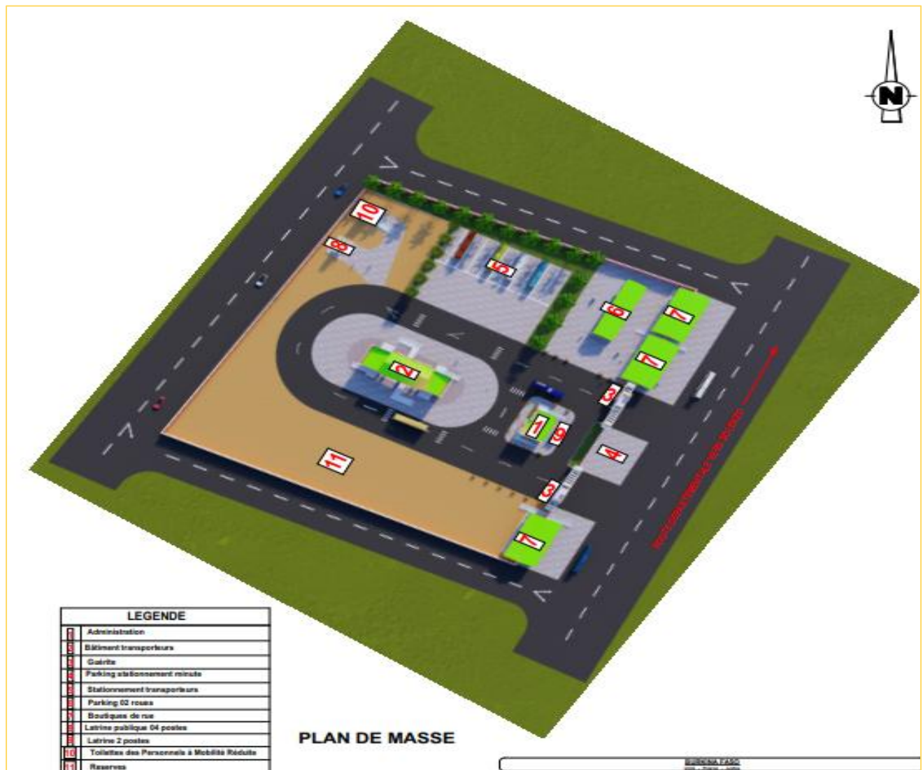
Carte 3: Plan de masse de la gare de Soin
